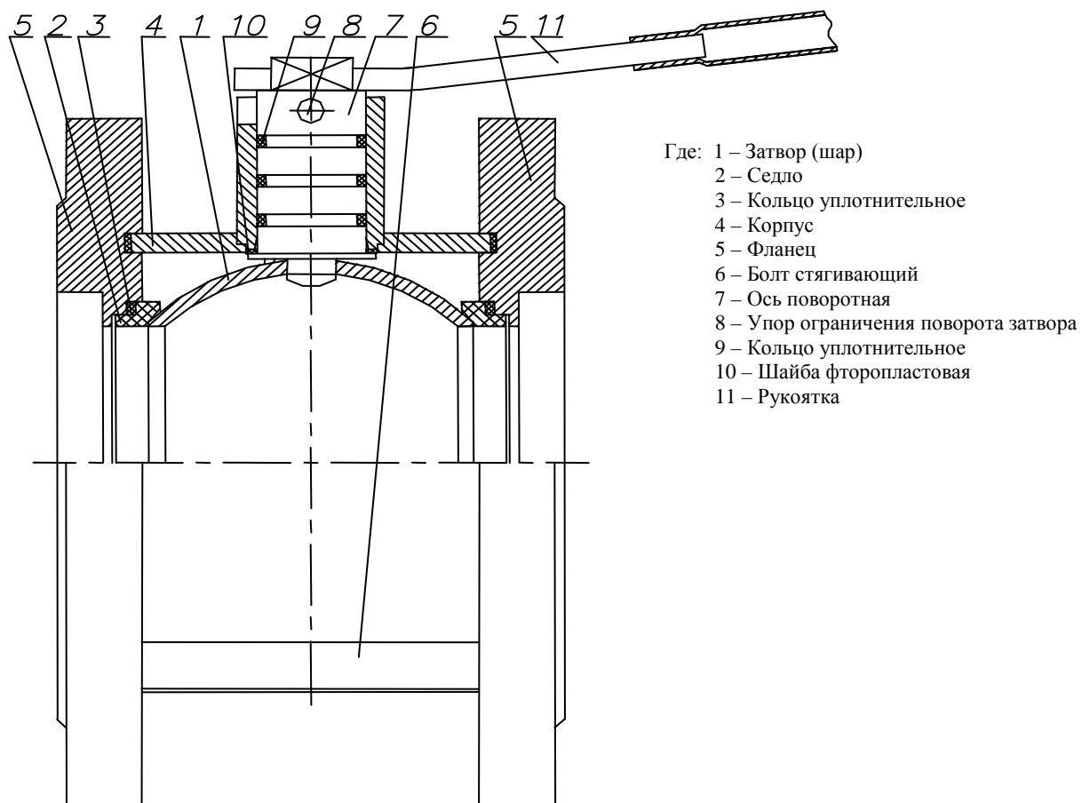
Рисунок 1. Общее устройство крана
